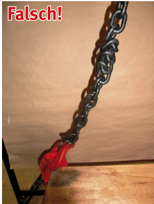
Bild 22-4: Stark verdrehte Kette. Beim Anheben der Last wird die Kette so beschädigt, dass sie nicht mehr weiter verwendet werden darf
