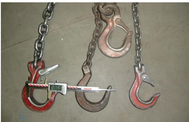
Bild 23-20: Die unteren drei Haken sind mehr als 10% geöffnet und damit ablegereif. 10% sind nicht viel! Aber trotzdem gefährlich!
