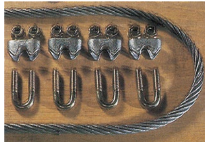
Bild 9-3: Mindestens 4 Seilklemmen sind nötig!
