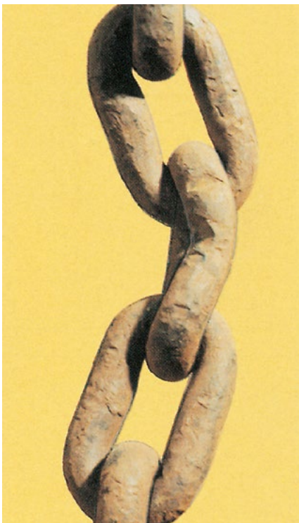
Bild 23-10: Kette mit verbogenem und eingekerbtem Kettenglied
