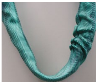
Bild 23-16: Durch Wärmeeinfluss zerstörte Ummantelung; Ablegereife auch wegen Sichtbarkeit der Einlage erreicht
